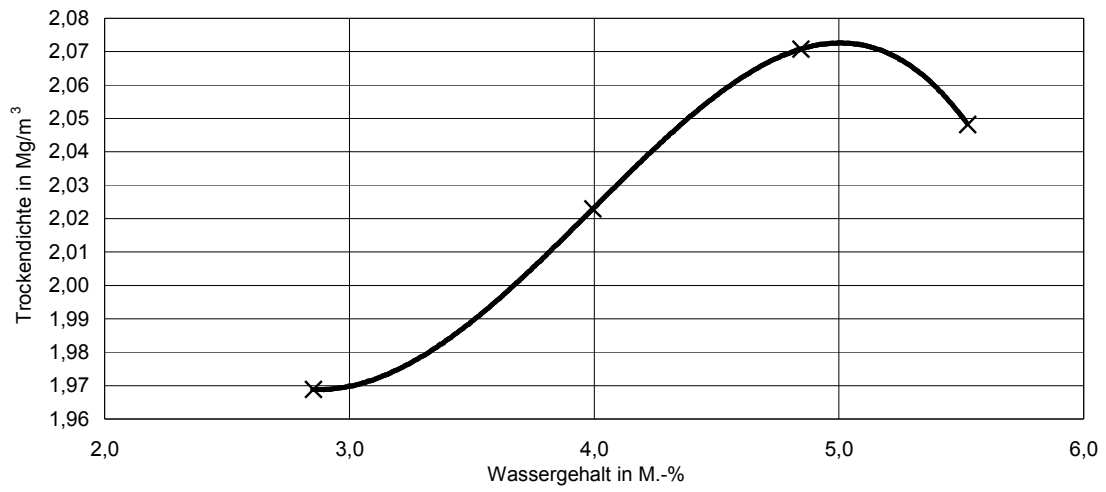
Proctorkurve des Baustoffgemisches 0/32 rd. (FSS) gemäß Prüfzeugnis Nr. 40680SoB/19 vom 11.12.2019
